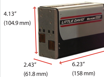
MicroJet HRP 1"
